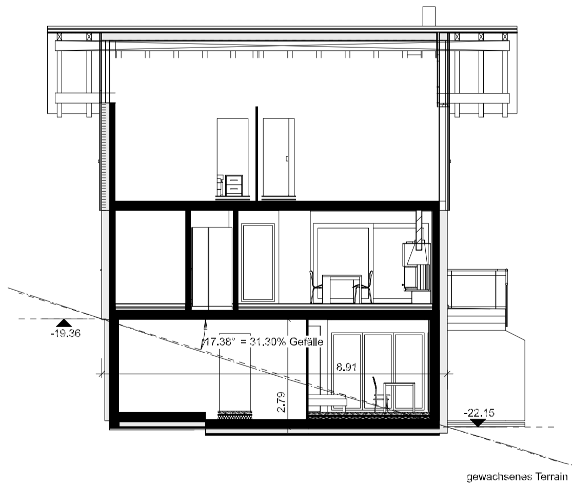
Hangneigung Nachweis
