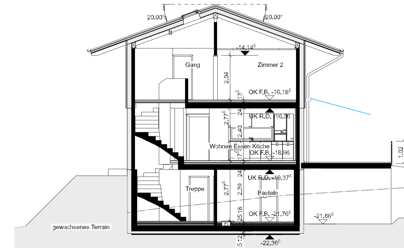
Schnitt B-B
