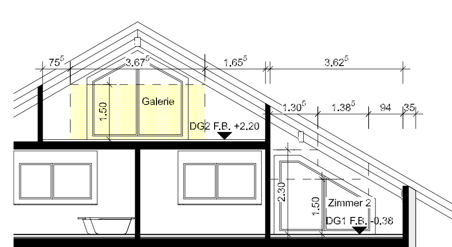
Schnitt Z33-Z30 Mindesthöhe nach BauV Art.67
