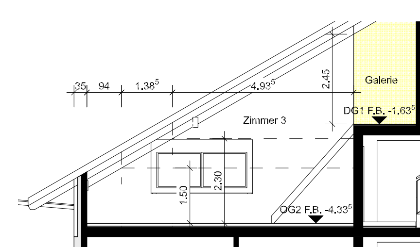
Schnitt Z30-Z30 Mindesthöhe nach BauV Art.67
