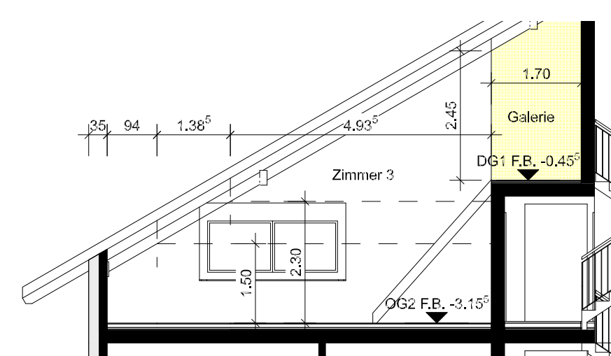
Schnitt Z32-Z33 Mindesthöhe nach BauV Art.67
