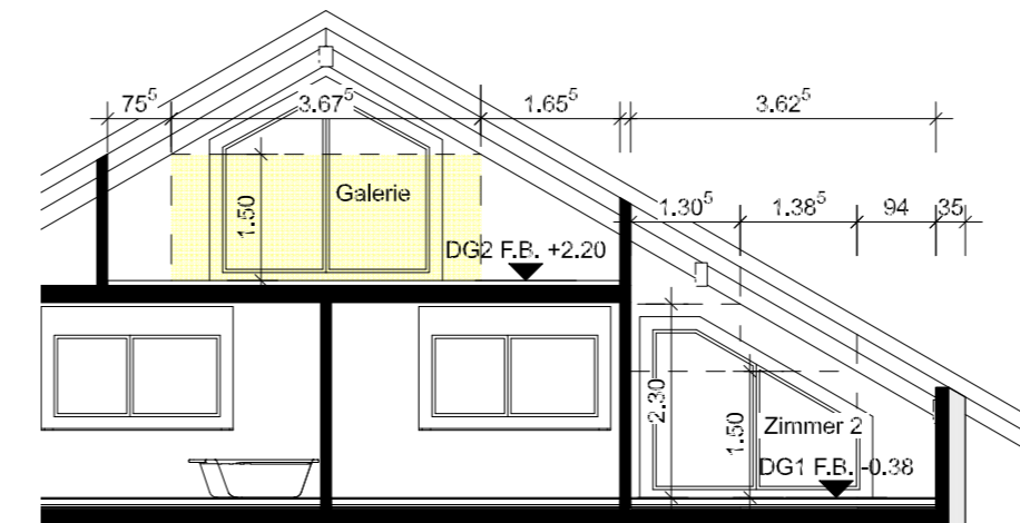
Schnitt Z33-Z33 Mindesthöhe nach BauV Art.67
