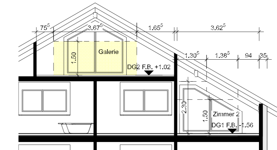
Schnitt Z31-Z31 Mindesthöhe nach BauV Art.67
